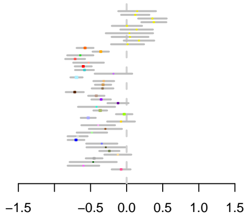
ENSG00000267508.1 SNP 2 only
