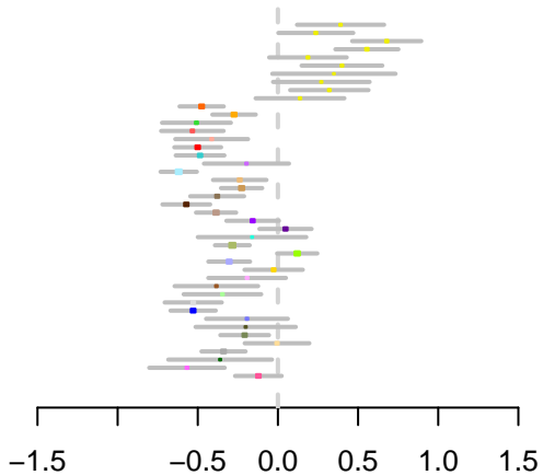
ENSG00000267508.1 SNP 1 only
